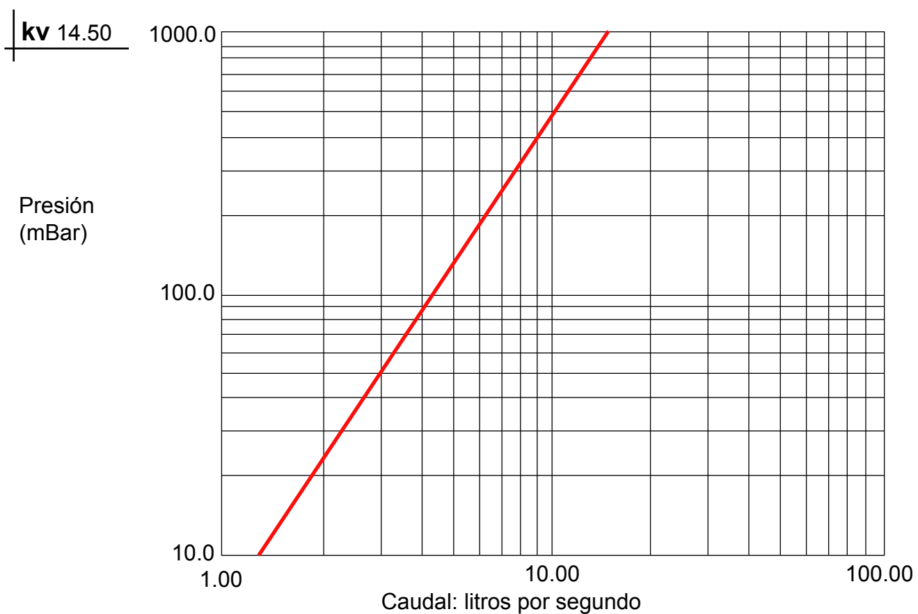
Diagrama 990844/TA/3: test de la pérdida de carga contra caudal del descalcificador magnético ELCLA5 Ø 2".
