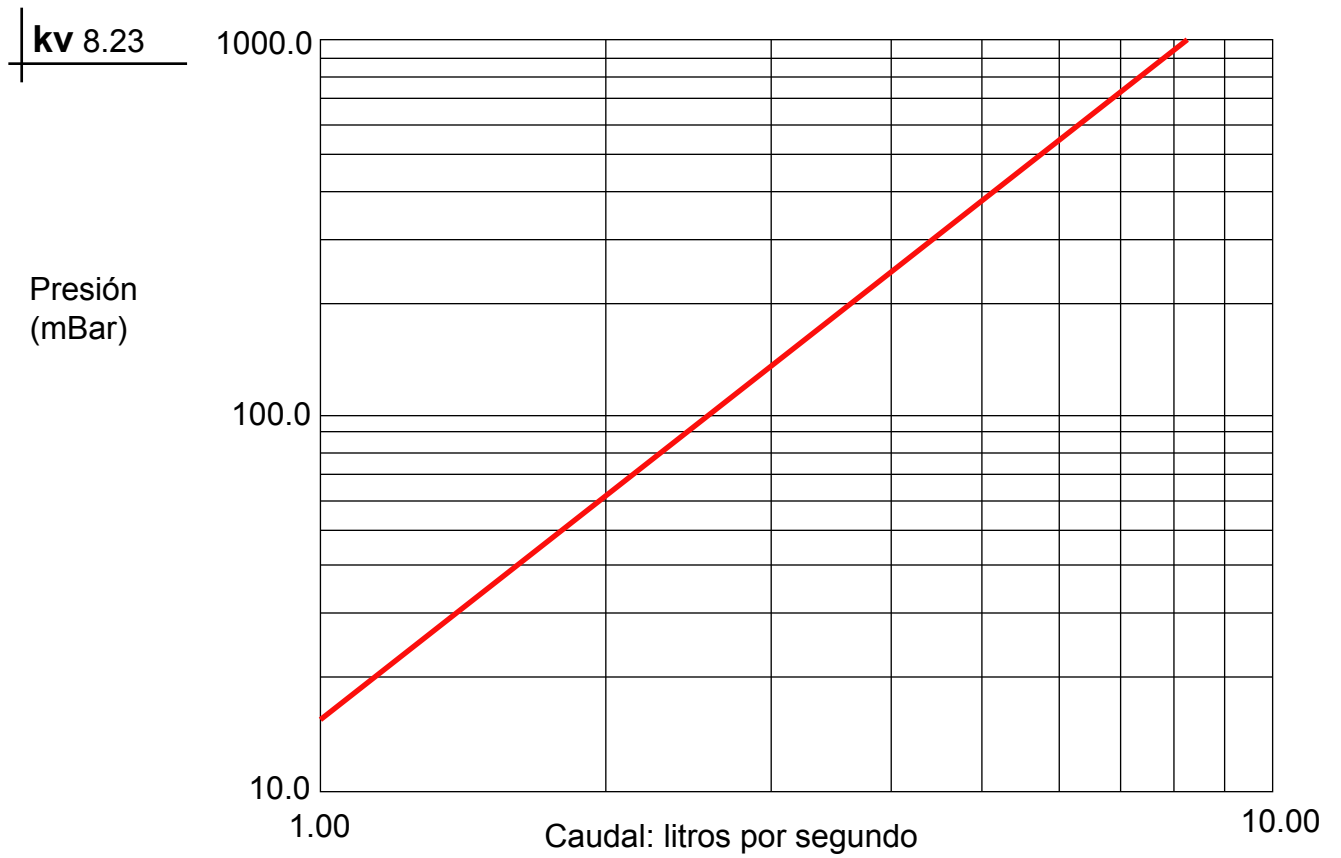
Diagrama 990844/TA/2: test de la pérdida de carga contra caudal del descalcificador magnético ELCLA4A Ø 1.1/2".
