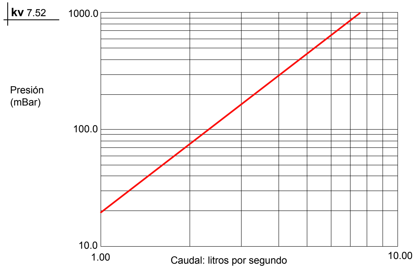
Diagrama 990844/TA/1: test de la pérdida de carga contra caudal del descalcificador magnético ELCLA4 Ø 1.1/4".
