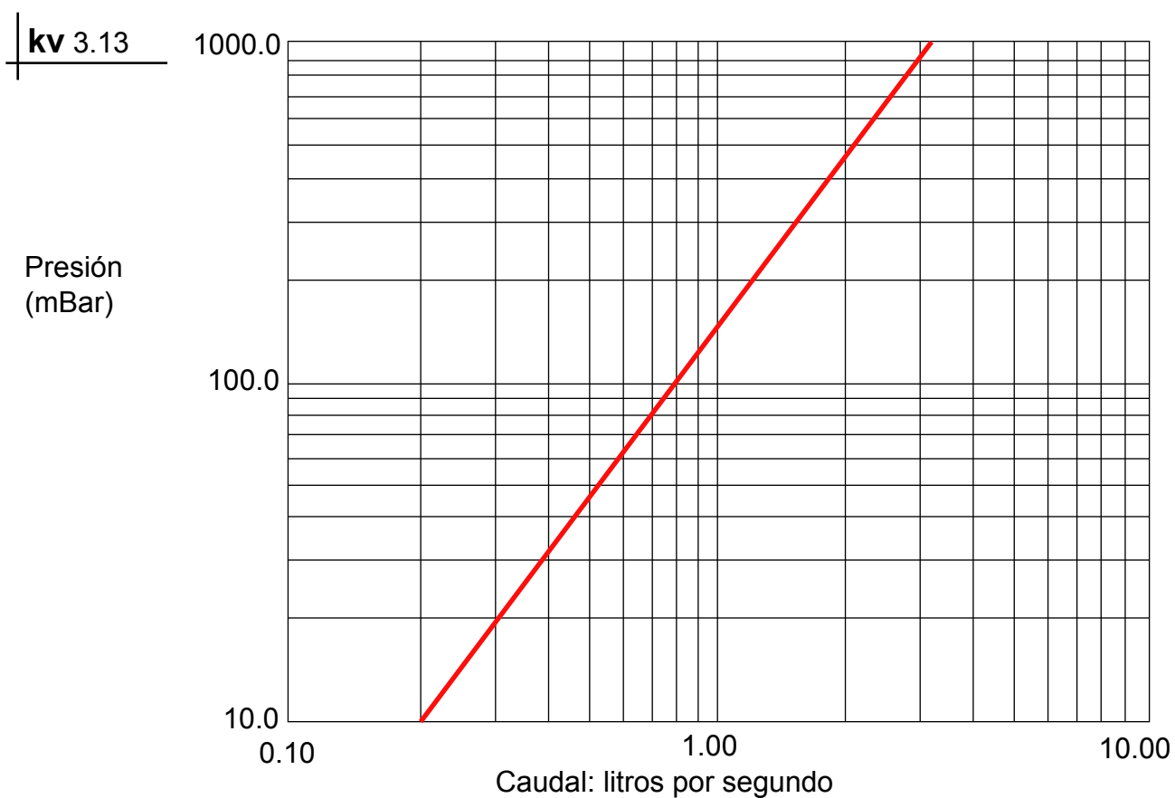
Diagrama 981559/4: test de la pérdida de carga contra caudal del descalcificador magnético ELCLA3 Ø 1".
