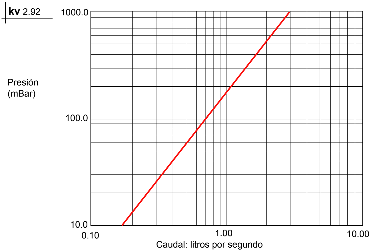
Diagrama 981559/3: test de la pérdida de carga contra caudal del descalcificador magnético ELCLA2 Ø 3/4".
