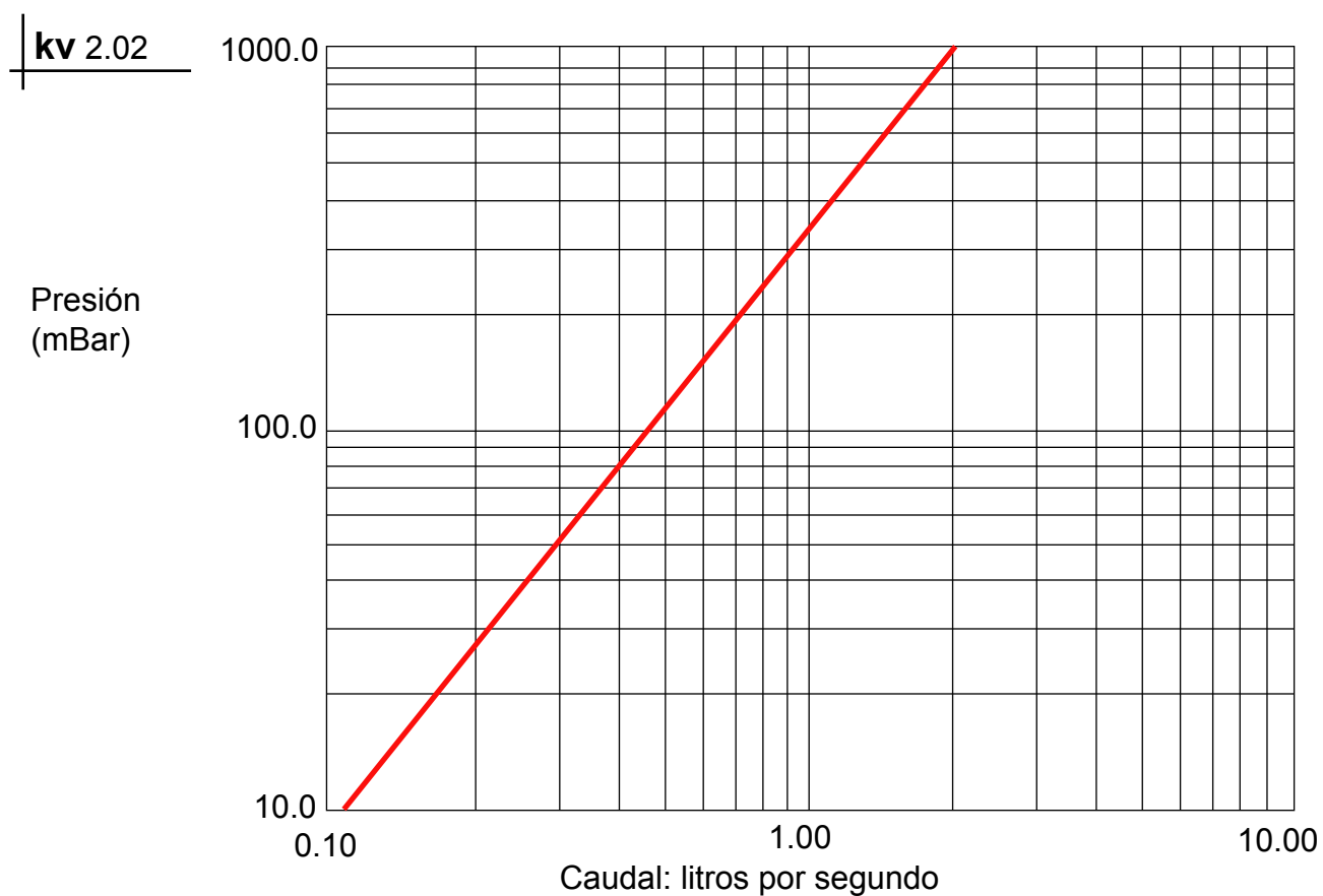
Diagrama 981559/2: test de la pérdida de carga contra caudal del descalcificador magnético ELCLA1 Ø 1/2".
