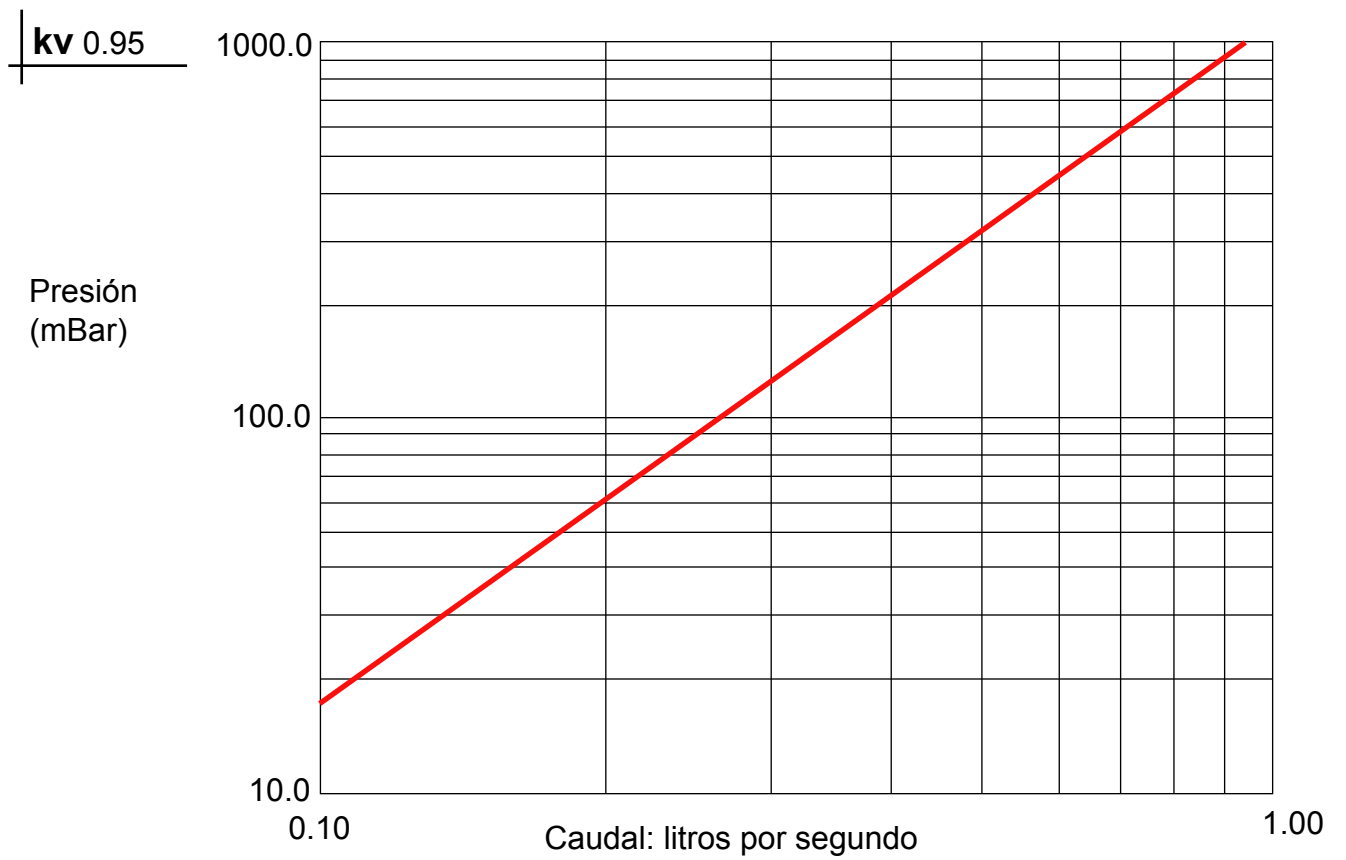
Diagrama 981559/1: test de la pérdida de carga contra caudal del descalcificador magnético MiniElcla Ø 1/2" y 3/4".
